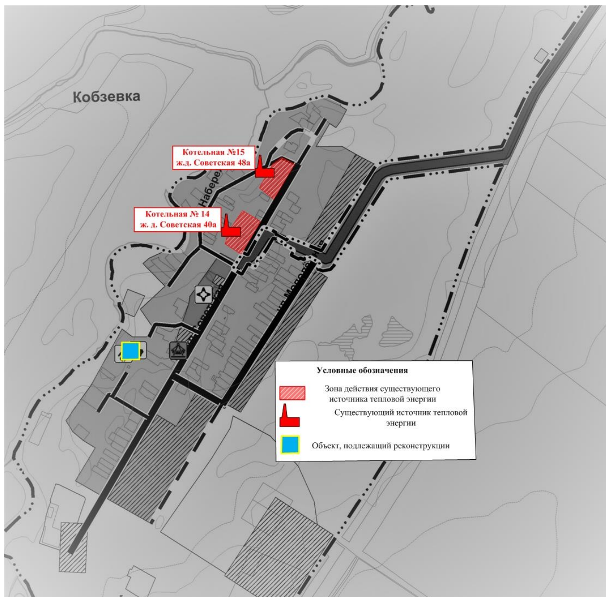
Рисунок 2.4.1 – Перспективные зоны теплоснабжения существующих котельных на территории п. Кобзевка
