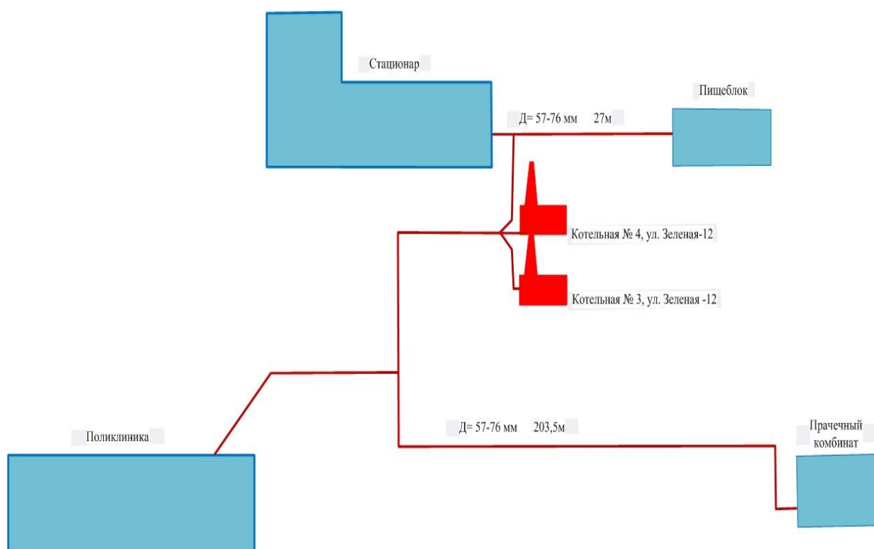
Рисунок 1.3.2.11-Принципиальная схема тепловых сетей Котельных МУ ЦМРБ м. р. Большеглушицкого района в селе Большая Глушица на улице Зеленой-12
