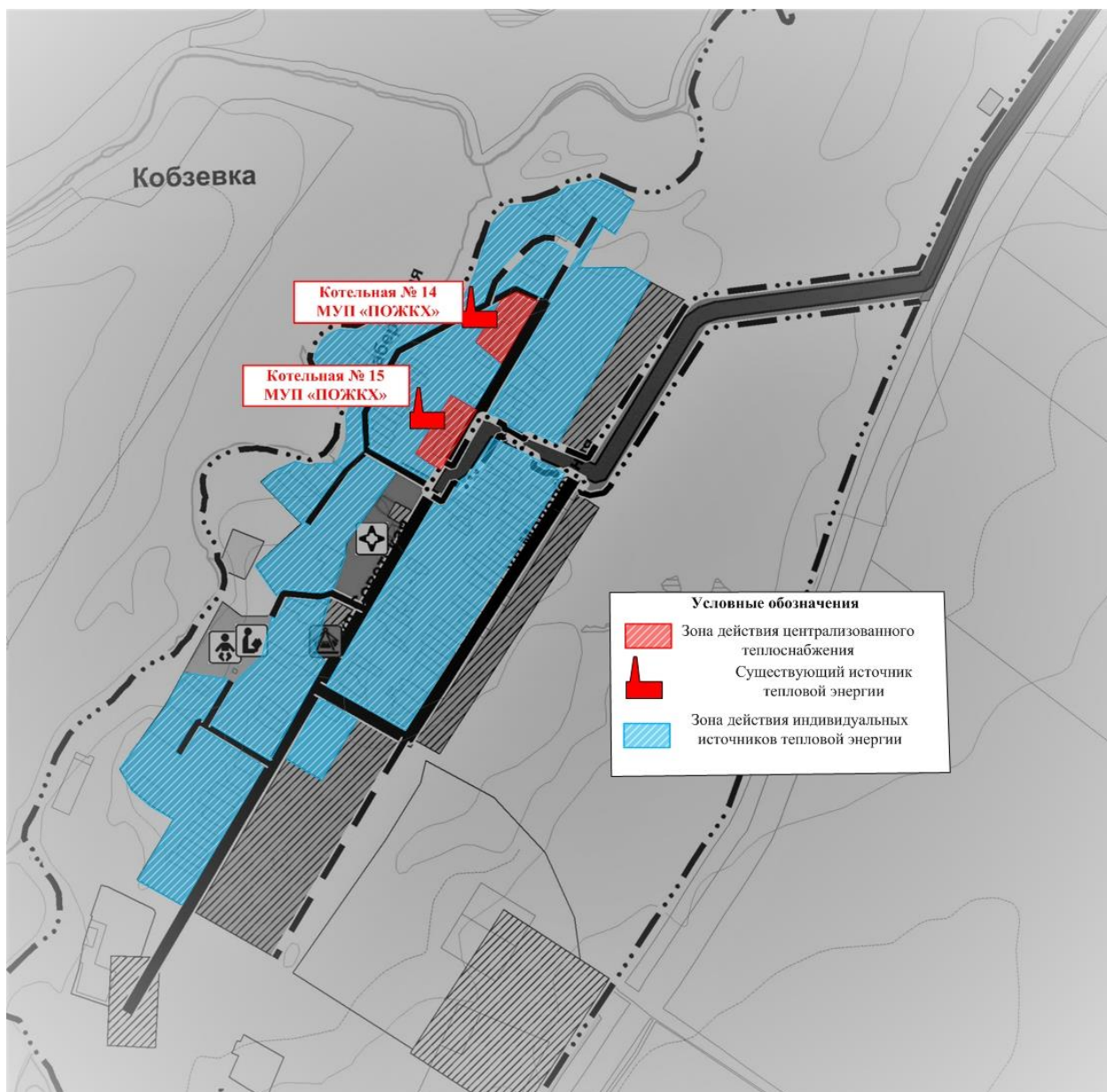
Рисунок 1.1.1.3 - Зоны действия централизованных и индивидуальных источников тепловой энергии на территории поселка Кобзевка
