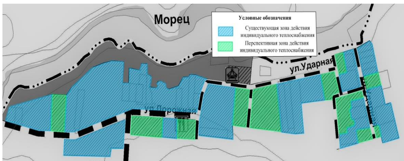
Рисунок 2.5.3 - Существующие и перспективные зоны действия индивидуального теплоснабжения на территории поселка Морец
